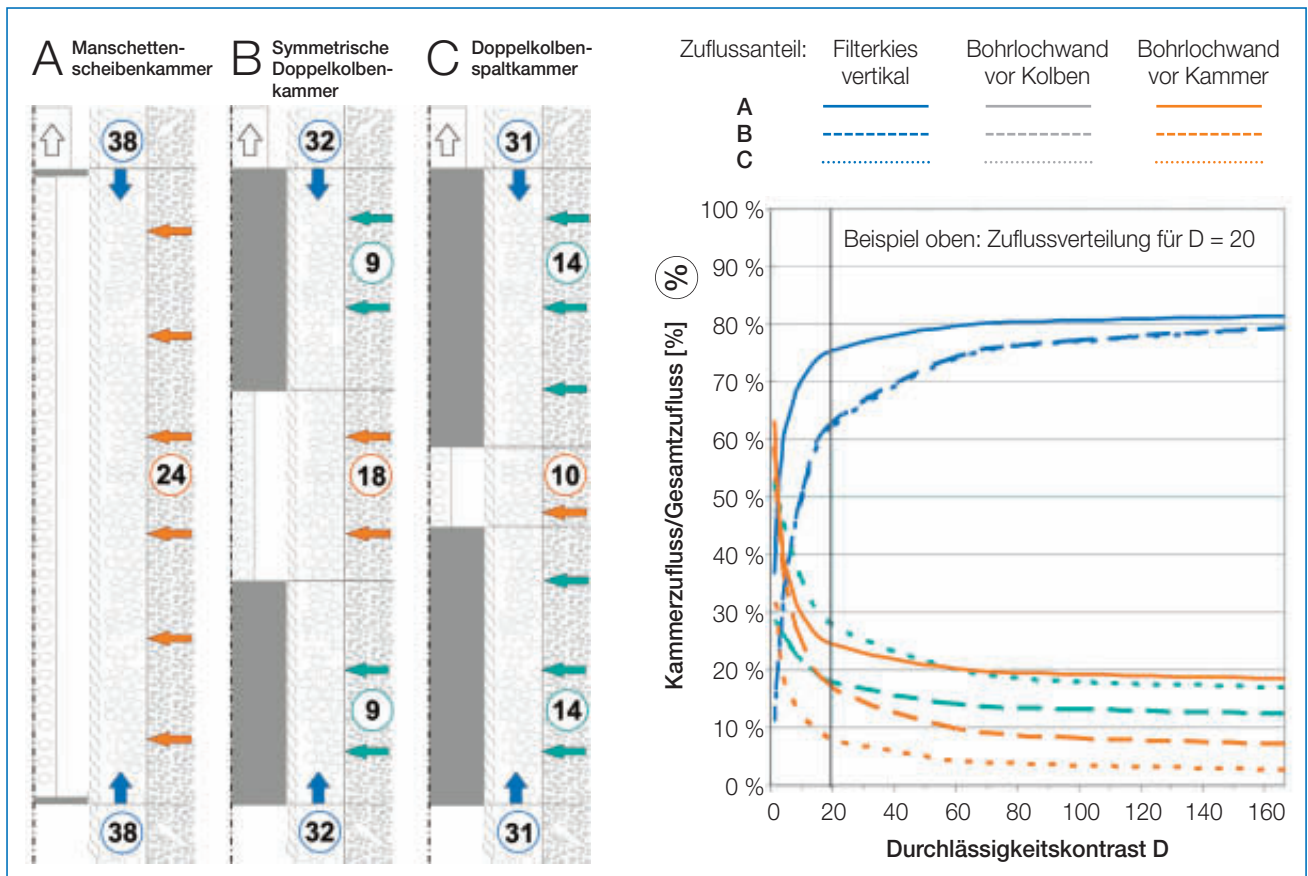
Abb. 3: Verteilung des Kammerzuflusses an (a) Manschettenkammer, (b) symmetrischer Doppelkolbenkammer und (c) Doppelkolbenspaltkammer für 1 < D < 167 und beispielhaft D=20
